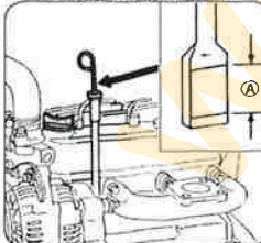
HET NIVEAU VAN DE THERMISCHE MOTOROLIE CONTROLEREN
